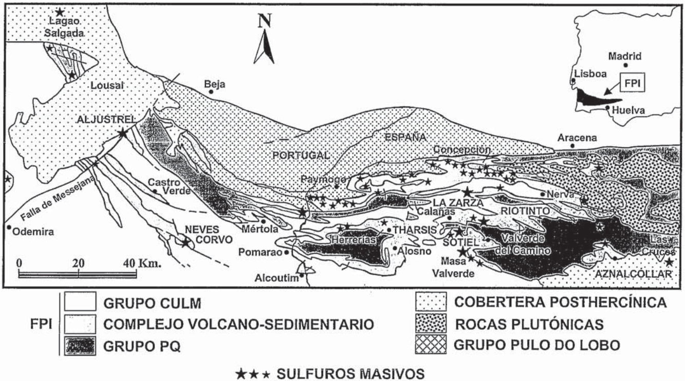
Fig. 1.- Mapa geológico regional de la Faja Pirítica Ibérica donde se muestra la localización de los principales depósitos de sulfuros masivos (modificado de Sáez et al., 1999).
