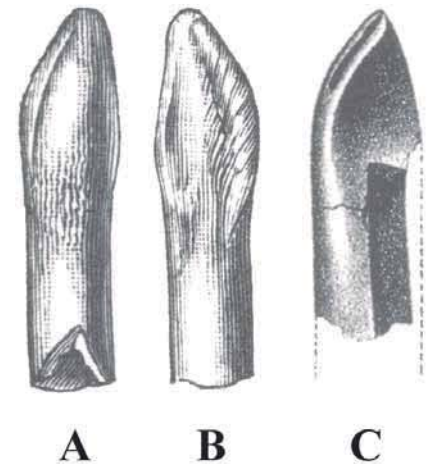
Fig. 2.- Dientes de Pleurocoelus nanus (A, B) y Astrodon johnstoni (C), en vistas labial (A) y lingual (B, C). A-B: tomado de Marsh (1896), C: tomado de Leidy (1865). Los dibujos no están a escala.
