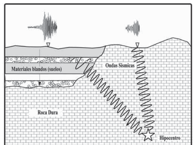
Fig. 1.- Esquema de paso de las ondas sísmicas en terrenos con distinta competencia
