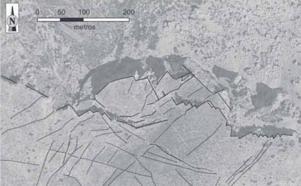
Fig. 3.- Fotografía aérea en la que se han cartografiado las principales fracturas existentes en el sector de las Simas de Partagat.
