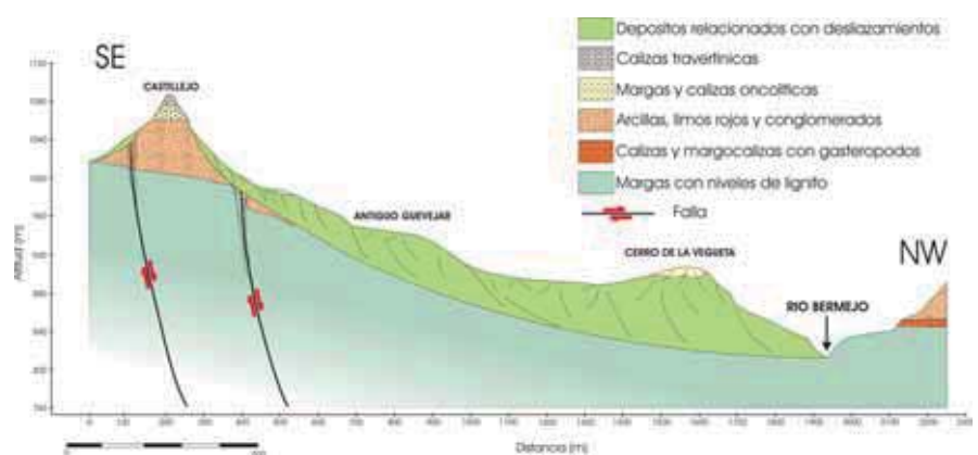
Fig. 3.- Corte geológico esquemático del deslizamiento de Güevéjar (véase localización en la Fig. 2).
