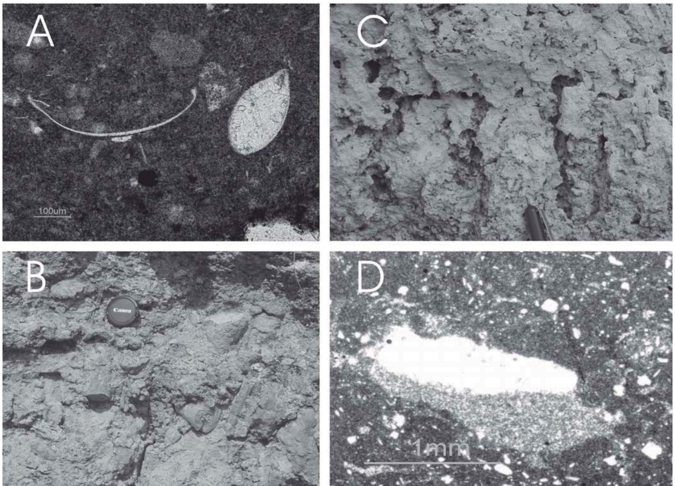
Fig. 2.- A) Caliza micrítica con ostrácodos (lámina delgada, nícoles cruzados); B) Toba (fitohermo) con moldes de tallos vegetales en caliza margosa; C) Rizolitos (moldes de raíces) en caliza palustre; D) Relleno de silt vadoso geopetal (lámina delgada, nícoles paralelos).
