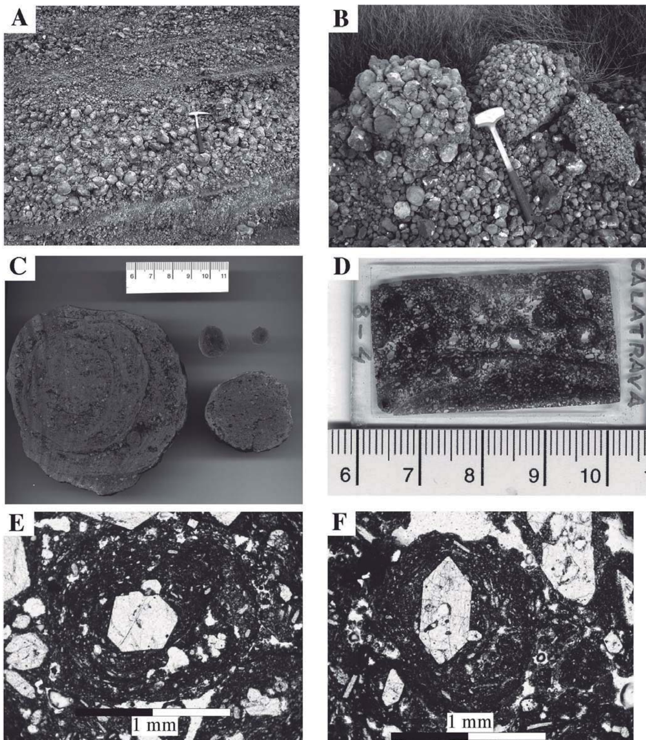
Fig. 1.- A) Modo de afloramiento de las tefras formadas por lapilli y bombas esferoidales del volcán Cabezo Segura (Ciudad Real). B) Bloques formados por lapilli y bombas esferoidales de diferentes granulometrías, cementados por calcita, desprendidos del afloramiento de la foto A. C) Secciones transversales de lapilli y bombas esferoidales de distinta granulometría, en los que es manifiesta su naturaleza clástica. D) Escáner de una lámina delgada de la bomba de la foto C, en la que se observan varios piroclastos esferoidales de tamaño lapilli, con diámetro \leq 4 mm. E y F) Lapilli esferoidal concéntrico (nícoles paralelos) que forma parte de la bomba esferoidal de la foto. Los fenocristales del núcleo son de olivino y los microfenocristales y microlitos dispuestos de forma concéntrica en torno a ellos son de olivino y clinopiroxeno.
