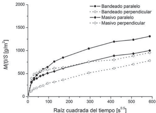
Fig. 4.- Absorción capilar del Travertino Clásico con facies bandeadas y masivas en la dirección paralela y perpendicular al bandeado.
