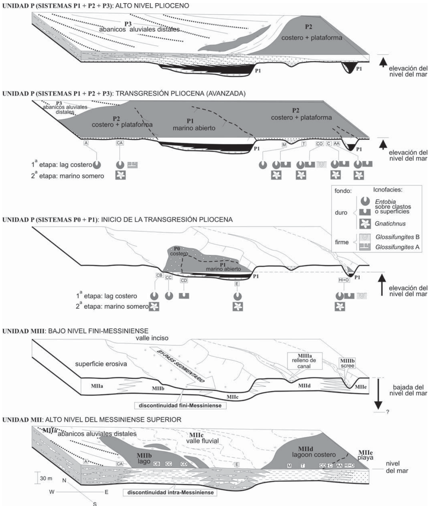
Fig. 2.- Esquemas que muestran la evolución paleogeográfica en distintos momentos del Messiniense superior y el Plioceno inferior. En los esquemas correspondientes al inicio y fase avanzada de la transgresión pliocena, se han representado las icnofacies registradas en cada sección.
