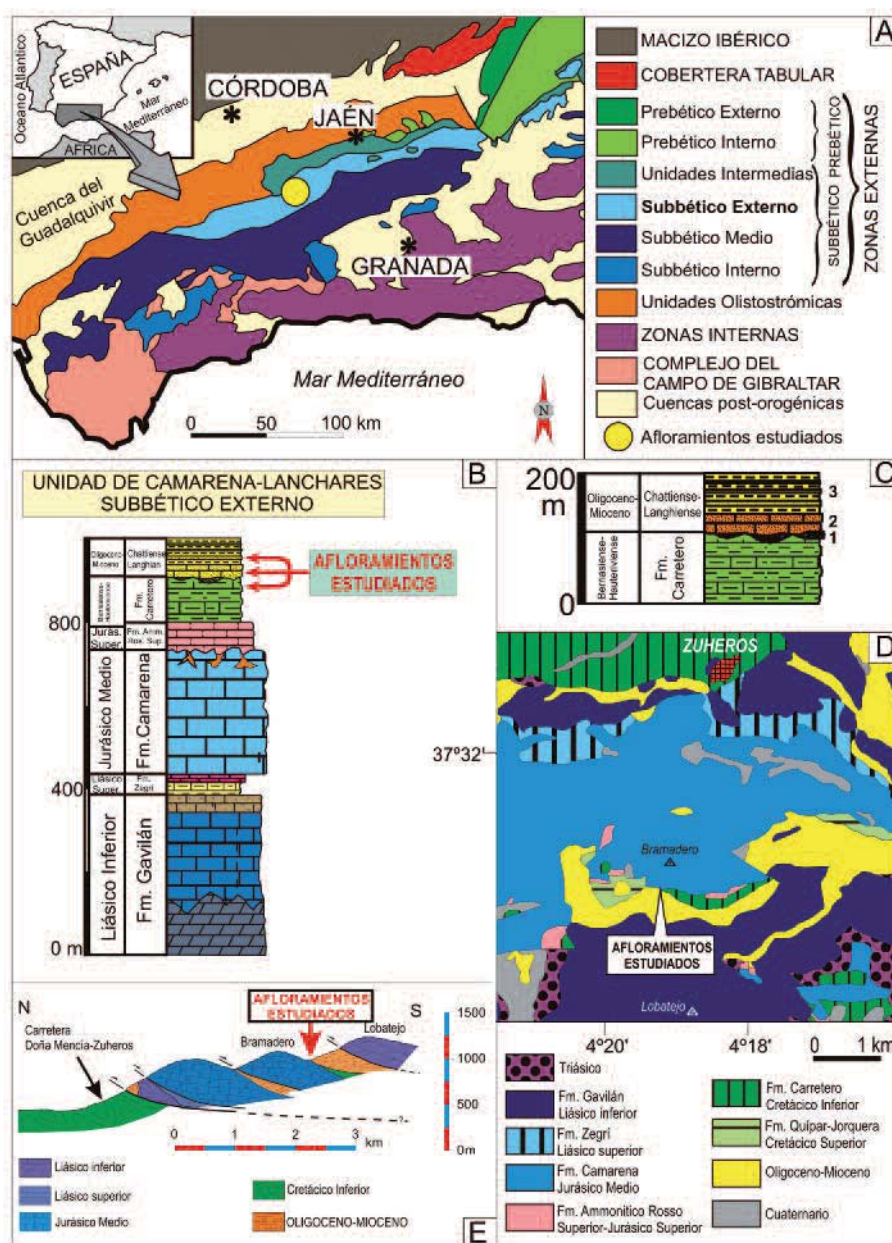
Fig. 1.- A) Situación geológica del área estudiada en el Subbético Externo de la Cordillera Bética. B) Columna estratigráfica de la Unidad de Camarena-Lanchares con la posición estratigráfica de los afloramientos estudiados. C) Miembros de la secuencia Cenozoica. D) Mapa geológico del sector estudiado. E) Corte geológico.
