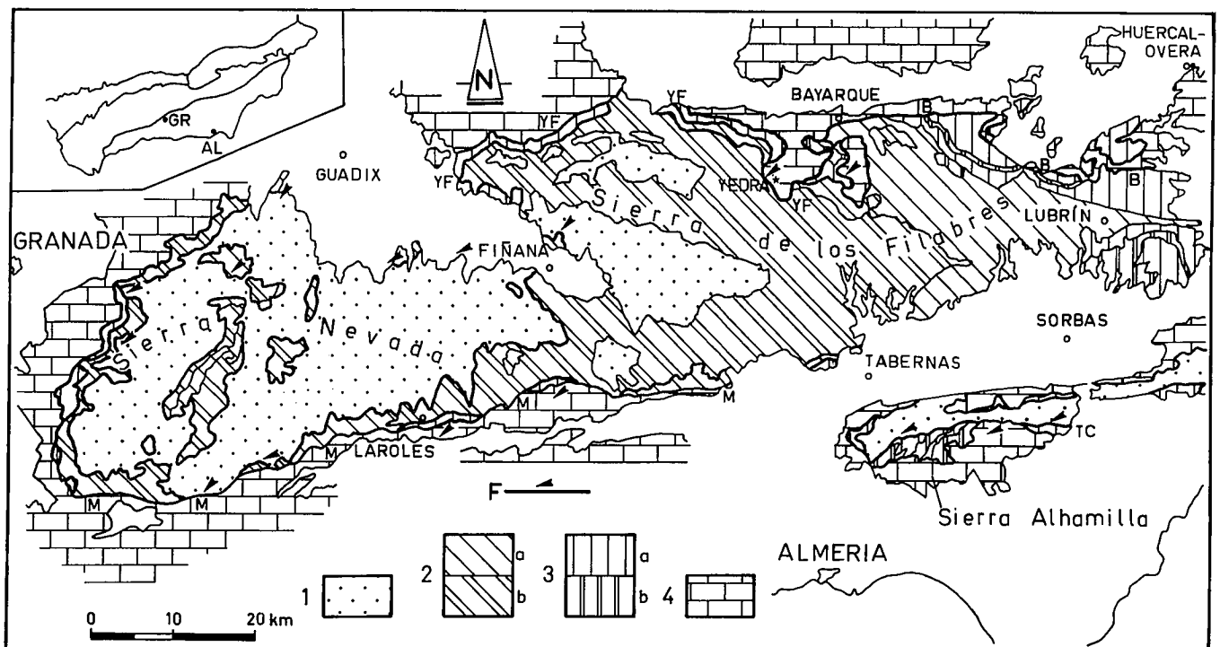
Fig. 1.—Esquema tectónico del Despegue Extensional de Filabres. 1) Unidad de Veleta. 2) Manto de Calar Alto (2a, Formación Tahal y Fm. Huertecica; 2b, Fm. Montenegro). 3) Manto de Bédar-Macael (3a, Fm. Tahal y mármoles de Atalaya; 3b, Fm. Montenegro). 4) Alpujárrides. F: Falla normal de bajo ángulo con indicación de sentido de movimiento (TC: Falla de Torres Cartas. M: Falla de Mecina; YF: Rampa de Yedra-Fiñana. B: Falla de Bayarque).
