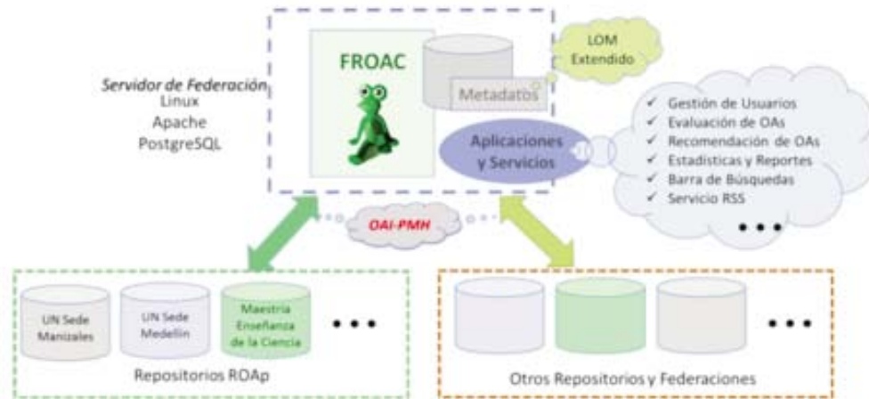
Figura 1. Modelo Federación de Repositorios de Objetos de Aprendizaje Colombia FROAC.
