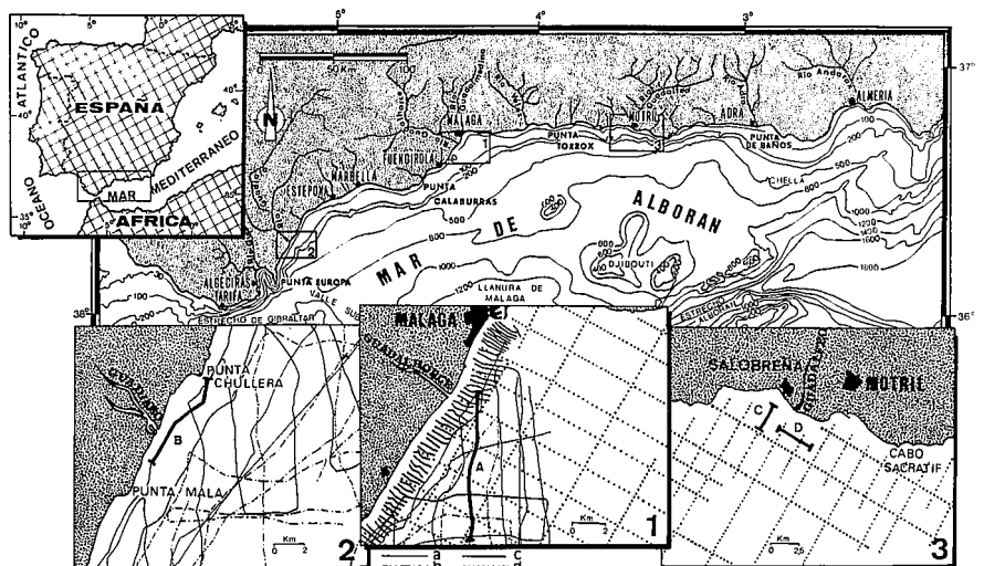
Fig.1.- Situación geográfica general del margen septentrional del Mar de Alborán, y del área del delta del Guadalhorce (1), área del delta del Guadiaro (2), y área del delta del Guadalfeo (3).
