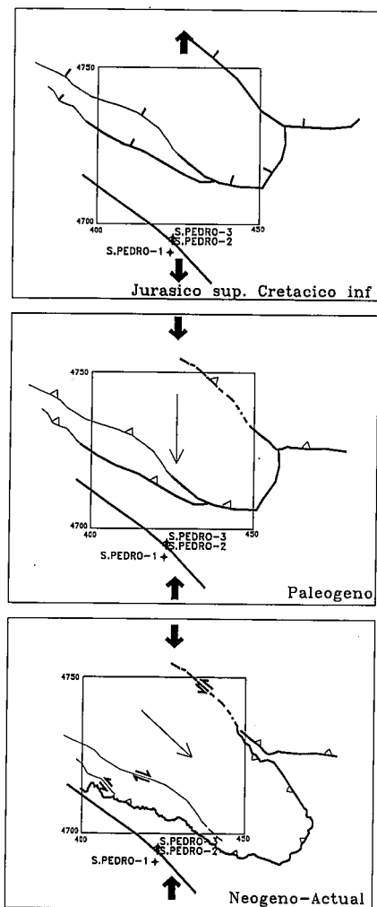
Fig. 5.— Esquema evolutivo del Arco de Rojas-Santa Casilda
