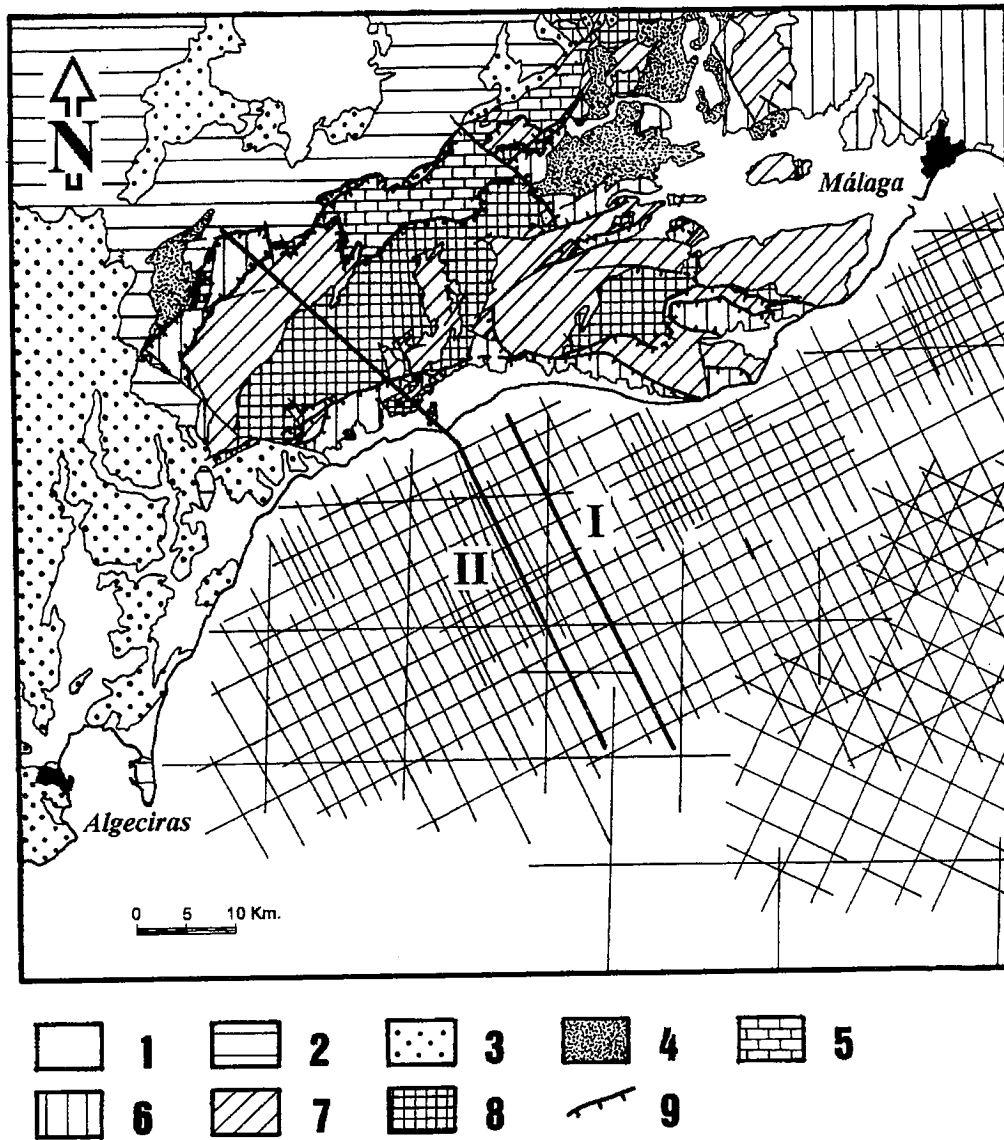
Fig. 1.- Situación de los perfiles de sísmica de reflexión considerados y contexto geológico regional. 1, Mioceno superior-Cuaternario; 2, Subbético; 3, Complejo de Flysch; 4, Complejo de Alosaina; 5, Complejo de la Dorsal; 6, Complejo Maláguide; 7, Complejo Alpujárride; 8, Unidades peridotíticas; 9, Principales fallas extensionales miocenas (desde el Burdigaliense superior); I, Localización del perfil sísmico de la figura 2; II, Localización del corte geológico de la figura 3. Modificado de Junta de Andalucía (1985), García-Dueñas y Balanyá (1991), y García-Dueñas et al. , (1992).
