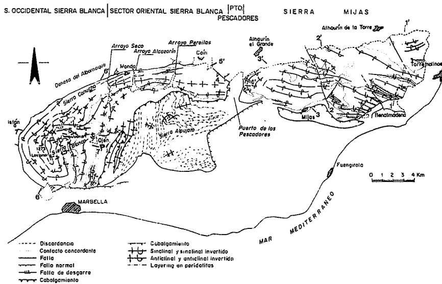
Fig. 2.- Mapa tectónico de las Sierras Blanca y Mijas. Los números indican la posición de los cortes hidrogeológicos de la figura 3.
