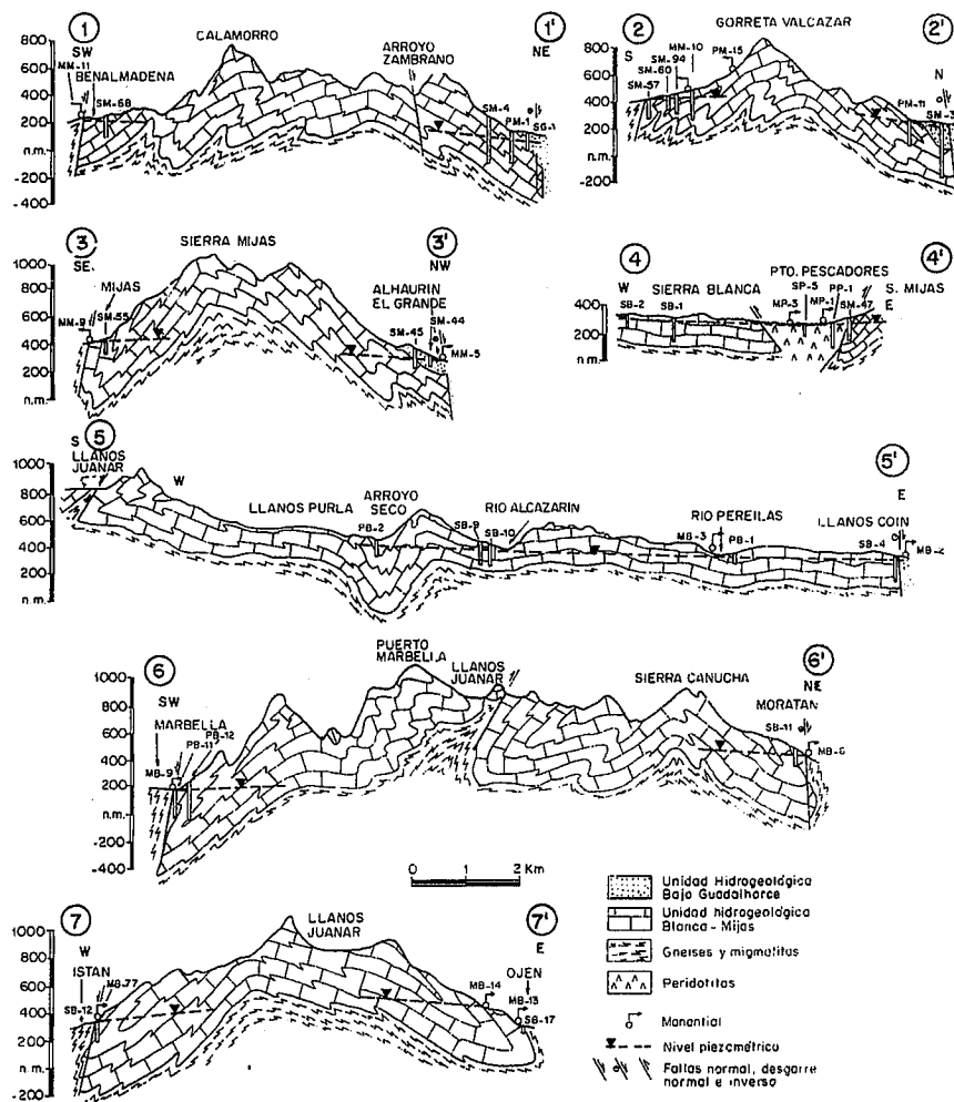
Fig. 3.- Cortes hidrogeológicos de las Sierras Blanca y Mijas.
