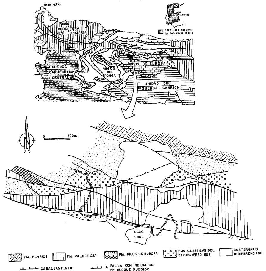
Fig. 1.- Situación geográfica y geológica del área de estudio.
