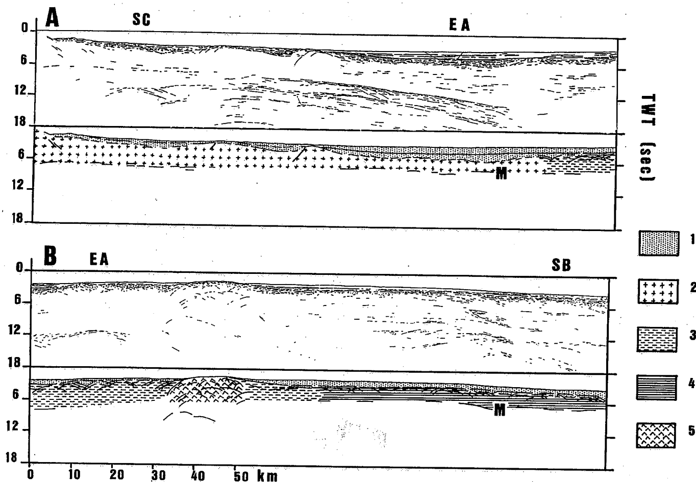
Fig. 3.- Interpretación de la estructura de la corteza, según la traza del perfil ESCI-Alborán 02. A) Esquema de los principales reflectores de el perfil ESCI-Alborán 02 y 02A, e interpretación de la estructura de la corteza según la traza de este perfil. B) Esquema de los principales reflectores de el perfil ESCI-Alborán 02B, e interpretación de la estructura de la corteza según la traza de este perfil. 1: Unidad sedimentaria; 2: Corteza continental adelgazada; 3: Corteza de transición; 4: Corteza oceánica; 5: Probable intrusión magmática; SC: Surco Central de Alborán; EA: Cuenca Oriental de Alborán; SB: Cuenca Surbalear; M: Discontinuidad corteza-manto. Localización en figura 1.
