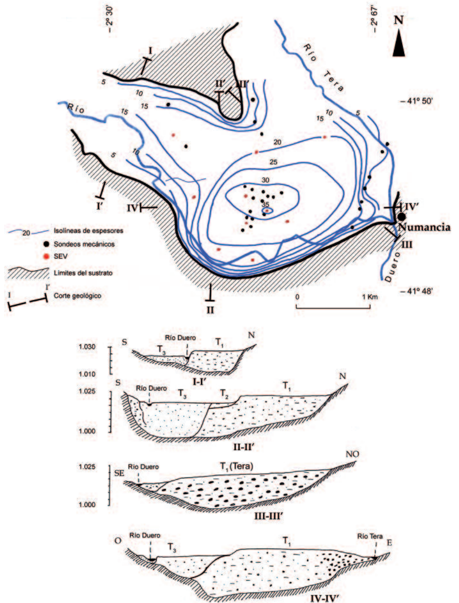
Fig. 3.- Espesores (m) del aluvial del Duero y Tera en Numancia. Cortes geológicos aproximados.
