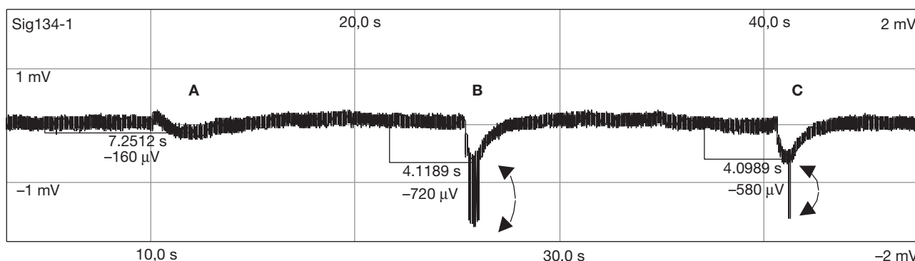
Figura 1. Respuestas típicas de EAG de C. welensii frente al ácido acético (A), ( E )-2-hexenal (B) y trementina (C). Las flechas indican anomalías en la señal, no consideradas en la medición de la respuesta.
