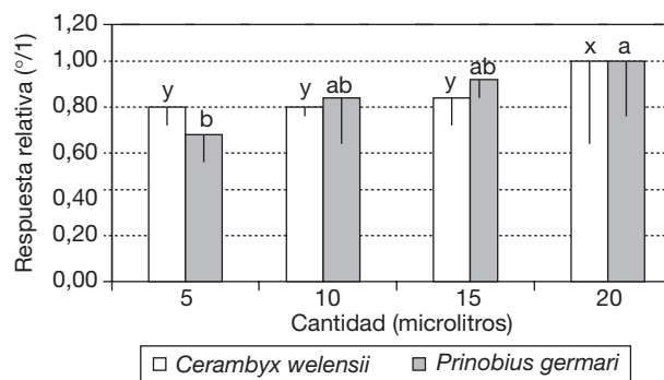
Figura 4. Respuestas netas de C. welensii y P. germari frente al estímulo estándar aplicado en distintas cantidades. La línea vertical muestra el intervalo de confianza al 95%. Letras distintas indican diferencias significativas al nivel 0,05.
