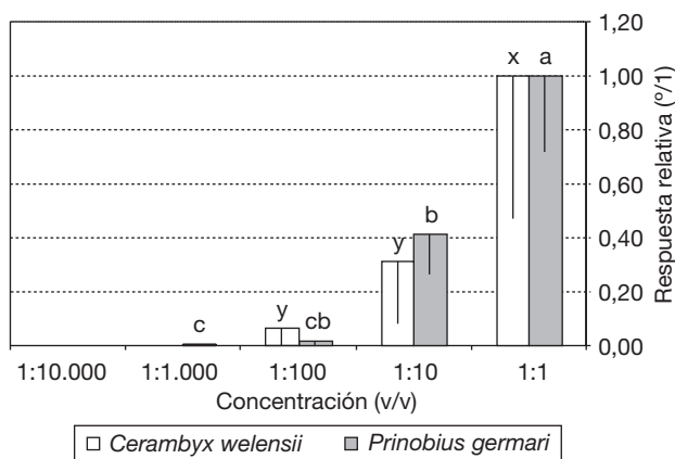
Figura 3. Respuestas netas de EAG de C. welensii y P. germari para distintas concentraciones del estímulo estándar. La línea vertical en el extremo de la barra muestra el intervalo de confianza al 95%. Letras distintas indican diferencias significativas.
