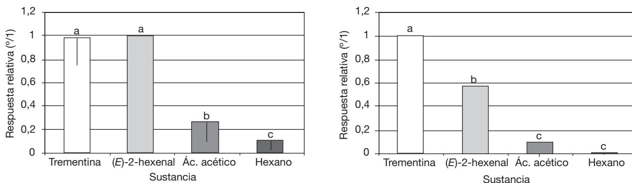
Figura 2. Respuestas relativas de EAG en C. welensii (izquierda) y P. germari (derecha) frente al ( E )-2-hexenal, trementina, ácido acético y el control de hexano. La respuesta relativa de C. welensii frente al ( E )-2-hexenal y de P. germari frente a la trementina es igual a 1. Las líneas en el extremo de la barra muestran la desviación típica. Letras distintas indican diferencias significativas en cada especie (prueba «t» de Student frente al valor \mu_0 = 100 y prueba de Wilcoxon entre pares de compuestos; ambas para un nivel de significación \alpha = 0,05 ).
