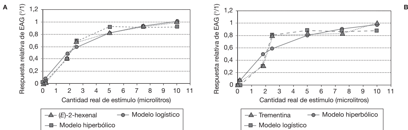
Figura 6. Variación de la repuesta de EAG de C. welensii (A) y P. germari (B) en función de las cantidades de estímulo estándar realmente aplicadas. Se reflejan los valores relativos respecto a la respuesta provocada por 20 \mu l de disolución 1:1 (v/v) (10 \mu l reales), así como dos modelos: logístico [ Y = a / (1 + e^{(b-cX)}) ; R^2 = 0,987 para C. welensii , y R^2 = 0,980 , para P. germari ] e hiperbólico [ Y = a * X / (b + X) ; R^2 = 0,984 para C. welensii , y R^2 = 0,930 para P. germari ].
