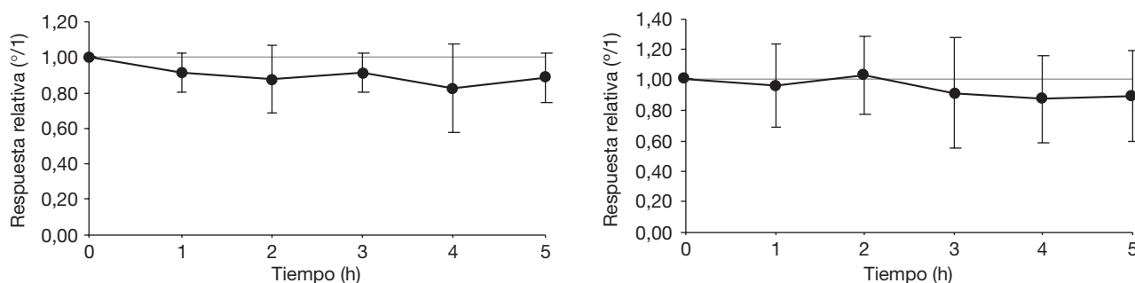
Figura 5. Variación de la respuesta relativa de C. welensii (izquierda) y P. germari (derecha) frente al estímulo estándar durante cinco horas (medias + desviación típica).
