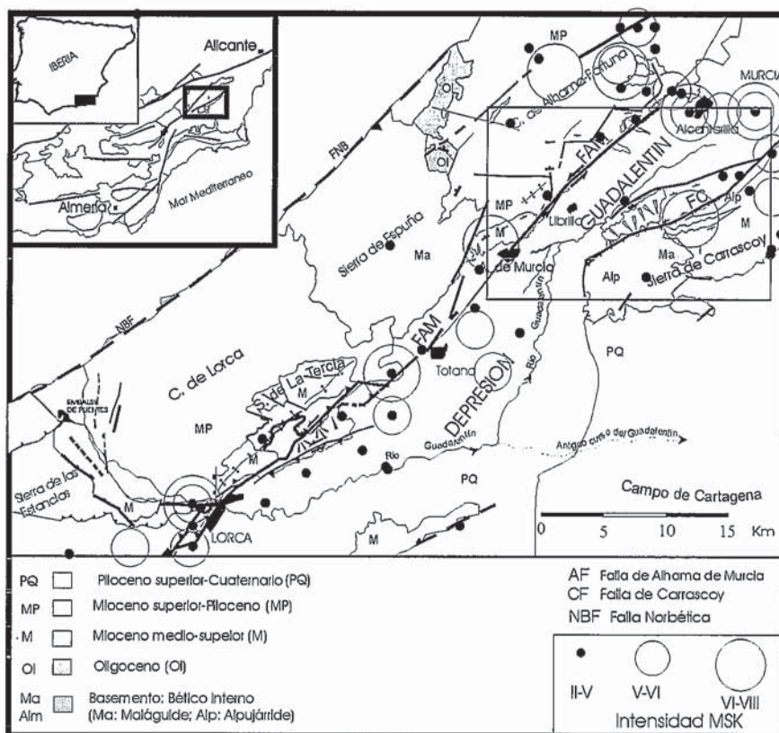
Fig. 1- Marco geológico de la Depresión del Guadalentín. Se representa en el recuadro la zona objeto del levantamiento gravimétrico, la Falla de Alhama de Murcia y la Falla de Carrascoy y la distribución de epicentros de los terremotos principales. Modificado de Martínez Díaz et al. , 2000.
