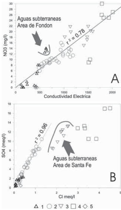
Fig. 4.- Distribución de los contenidos en NO 3 - con respecto a la conductividad eléctrica de las aguas y Cl - con respecto a los contenidos en SO 4 2- . Se han separado los grupos señalados en el texto, correspondientes a las aguas superficiales (1: área de cabecera, 2: área central, 3: área final) y a las aguas subterráneas (4: acuífero detrítico 5 acuífero carbonatado).
