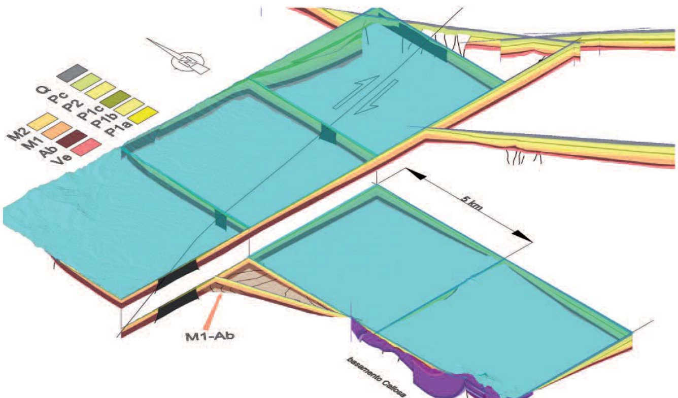
Fig. 3.- Modelo geológico 3D de la Cuenca del Bajo Segura. En primer término se muestra la superficie entre los sintemas Ab y M1.
