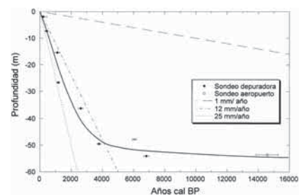
Fig. 2.- Relación entre la profundidad (respecto al nivel del mar actual) y el promedio del intervalo de la edad calibrada BP (datos en Tabla I). Las líneas rectas discontinuas representan tasas ficticias de sedimentación constante (1, 12 y 25 mm/años). La línea continua muestra la tendencia general de la tasa de sedimentación deducida para Pleistoceno superior y Holoceno del Delta del Llobregat.
