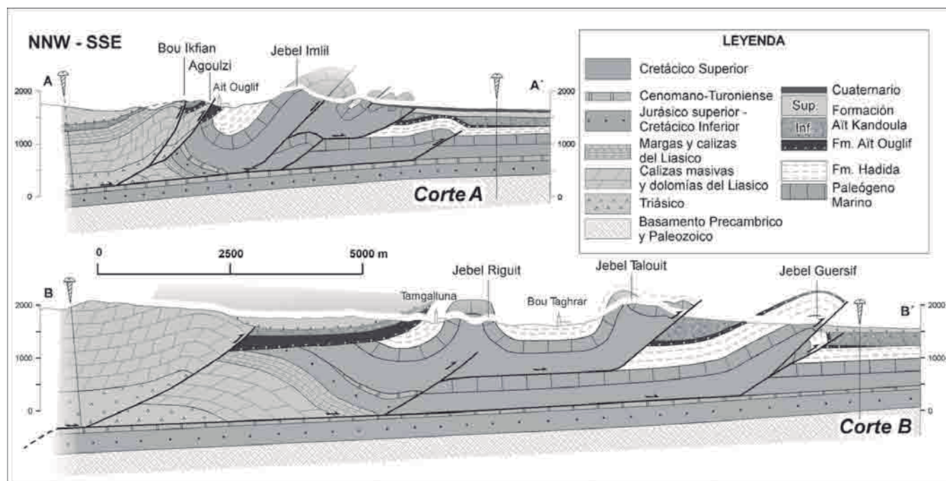
Fig. 3.- Cortes geológicos que muestran la estructura geológica de la Zona Sub-Atlásica en el sector estudiado.
