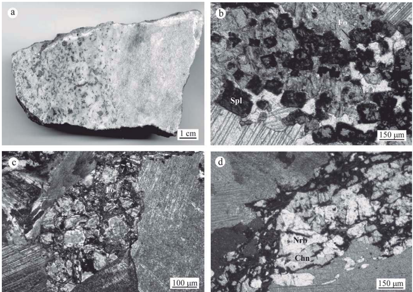
Fig. 2.- (a) Mármol dolomítico con niveles de tamaño de grano grueso que contienen la asociación condroditita y/o norbergita-espínela-magnetita; (b) cristales idiomorfos de espínela verdosa con forsterita completamente serpentizada en matriz dolomítica, tomada con nicoles paralelos; (c) Cristal de forsterita serpentizada; (d) Relación textural de la condroditita y la norbergita; (c) y (d) tomadas con nicoles cruzados.
