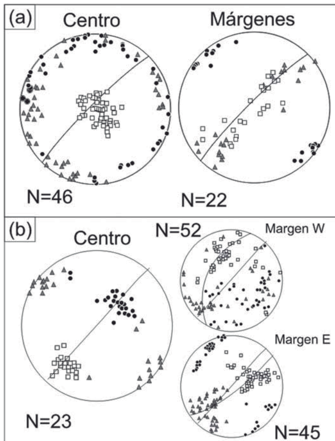
Fig. 3.- Estereogramas de ejes de susceptibilidad magnética para las estaciones (A) COR-03 y (B) FLW-05 distribuidos por sectores (centro y márgenes).
