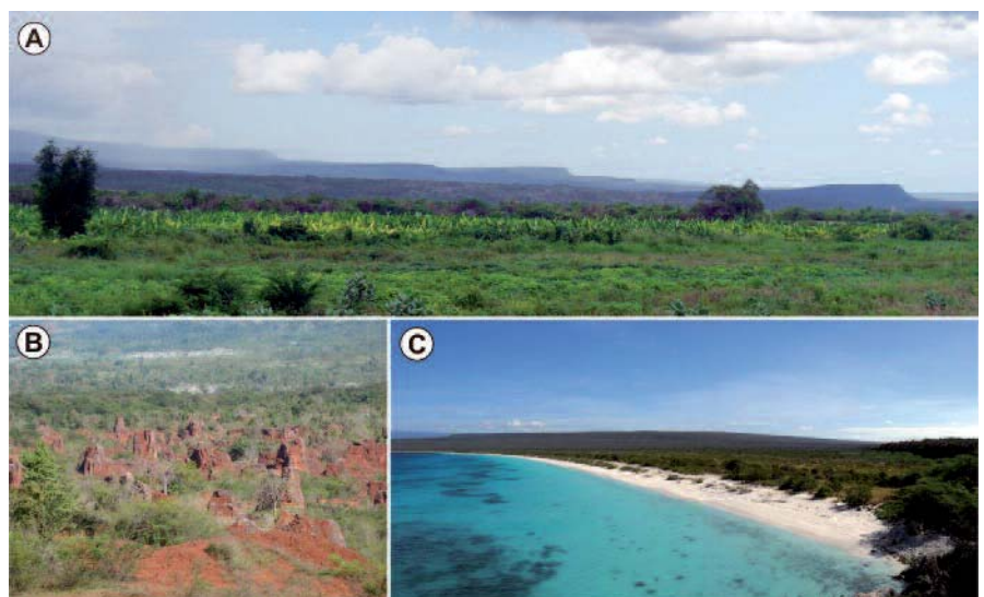
Fig. 2.- Fotografías de algunos Lugares de Interés Geológico en la Península de Bahoruco. A. Paleoescarpes del P. N. Jaragua. B. Minas de bauxita de Las Mercedes. C. Bahía de las Águilas. Fig. 2.- Pictures of some of the proposed geosites for the Bahoruco peninsula. A: Palaeoscarps in the P.N. Jaragua. B: Las Mercedes bauxite mine. C: Las Águilas Bay.
