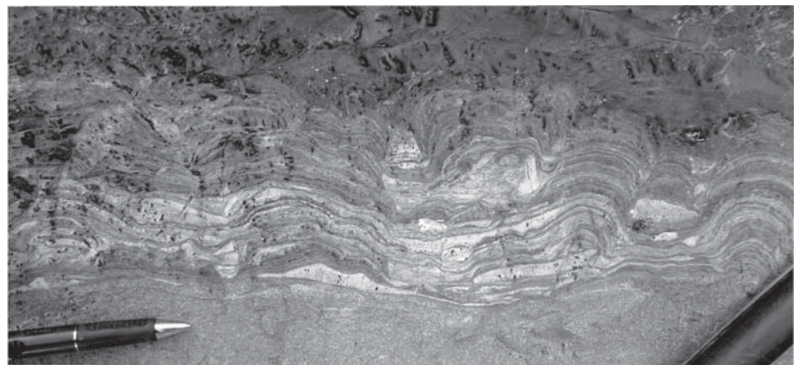
Fig. 4.- Fotografía de afloramiento de los estromatolitos cómicos de la Asociación de Facies 3 tapizando un nivel de grainstone oolítico (parte inferior). Lápiz como escala.
