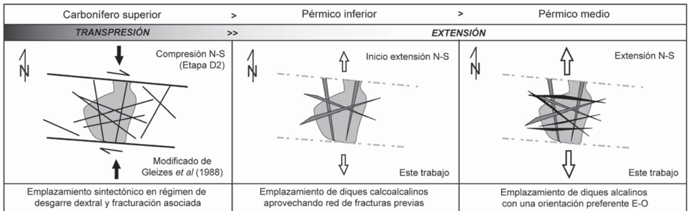
Fig. 5.- Modelo conceptual (en planta) del emplazamiento de los diques de lamprófidio del Plutón de Panticosa en relación al escenario dinámico en el intervalo Carbonífero superior - Pérmico inferior. Explicación en el texto.
