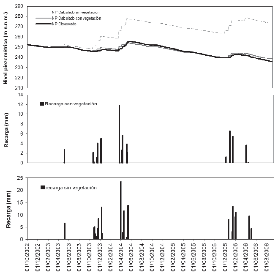
Fig. 2.- Comparación de las variaciones piezométricas reales con las obtenidas a partir del drenaje profundo resultado de la aplicación HYDROBAL con y sin vegetación.
