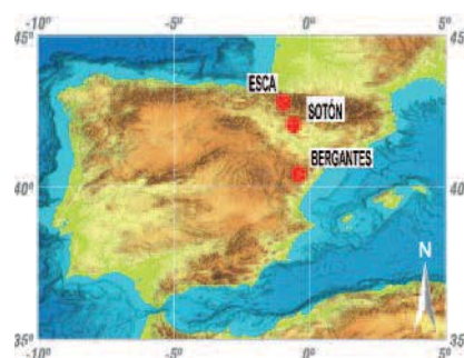
Fig. 1.- Situación de cuencas en SRTM30.
