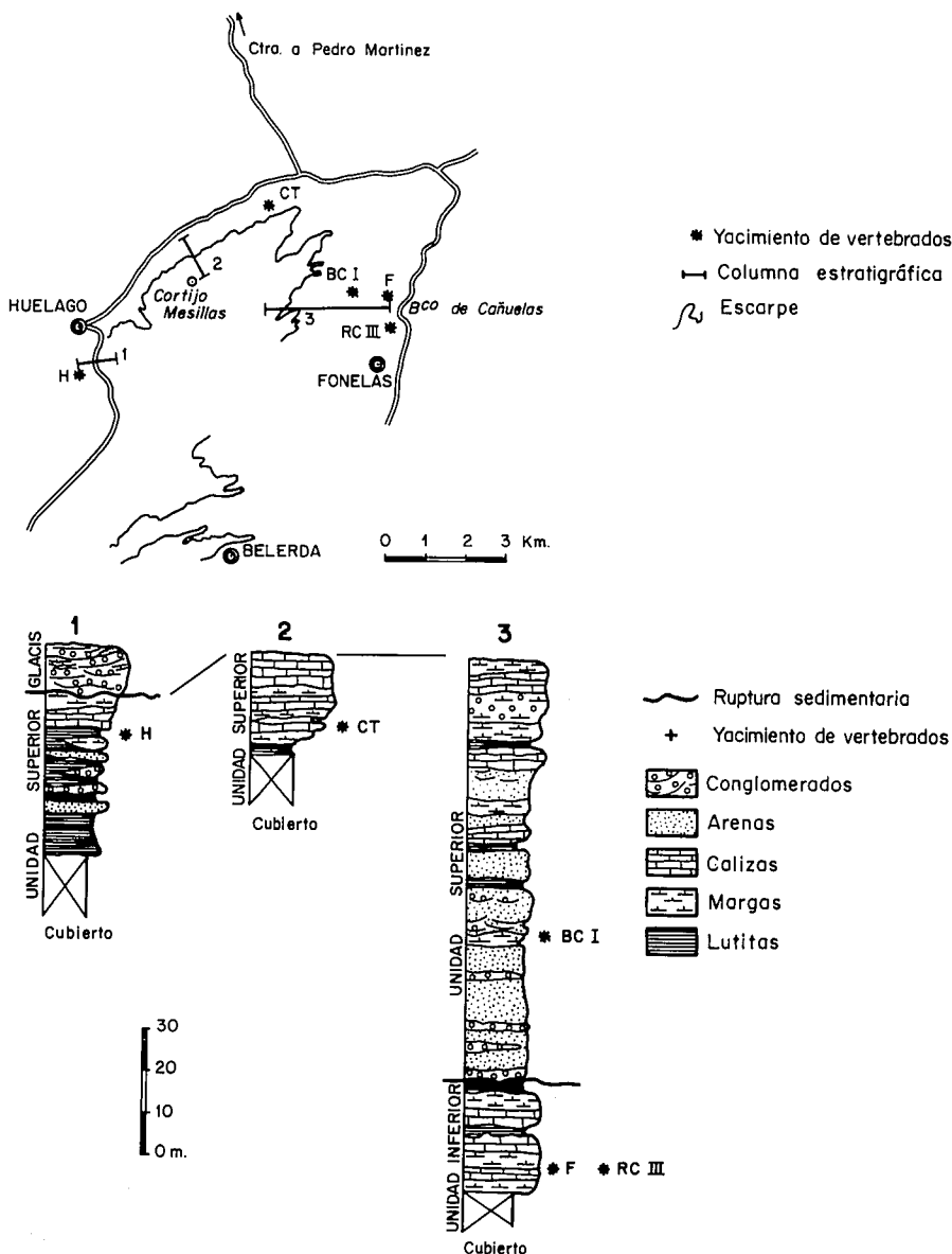
Fig. 1.—Situación geográfica y representación gráfica de los yacimientos y columnas estratigráficas más significativas. La columna núm. 1 corresponde a la serie de Huélago, la núm. 2 a la serie del Cortijo de las Mesillas y la núm. 3 a la del Barranco de Cañuelas. Abreviaturas de los nombres de los yacimientos: H=Huélago; CT=Cortijo de Tapia; BCI=Barranco de Cañuelas I; F= Fonelas; RC=Rambla del Conejo III.
