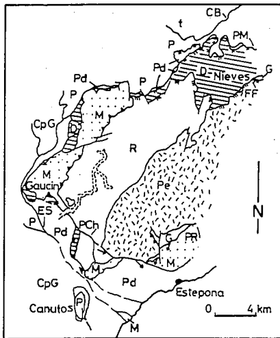
Fig. 1.—Esquema del contacto Dom. Alborán-Dom. Sudibérico al W y S de Ronda. Las flechas representadas indican el movimiento del bloque de techo. P: Penibético (t: Triás); CpG: Flyschs Campo de Gibraltar; Pd: Predorsal; D: Dorsal; M: Maláguide; R: M. de los Reales (Pe: peridotitas); G: M. de Guadaiza. Fallas o zonas de falla: Cabrejas (CB), Pompeya (PM), Fuenfría (FF), Piedras Recias (PR), Pto. Chamorro (PCh) y Espartina (ES).
