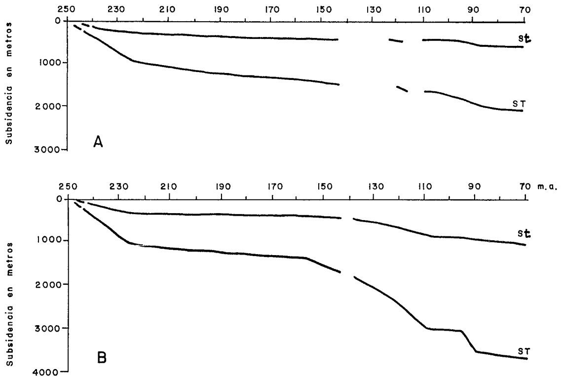
Fig. 3.—Relación entre la Subsidencia tectonotérmica y el tiempo: St - t . A: Triásico y Jurásico. B: Cretácico. Línea continua: Rama Castellana. Línea discontinua: Rama Aragonesa.
