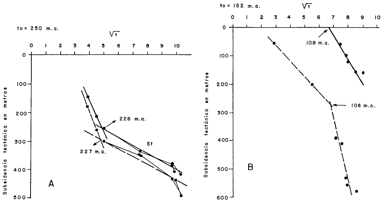
Fig. 2.—Curvas de subsidencia en la Rama Castellana (A) y en la Aragonesa (B) de la Cordillera ibérica. S_T : Subsidencia total. S_T : Subsidencia tectonotérmica. (Escala cronológica: Geological Time Scale de la Geological Society of America, 1983.)
