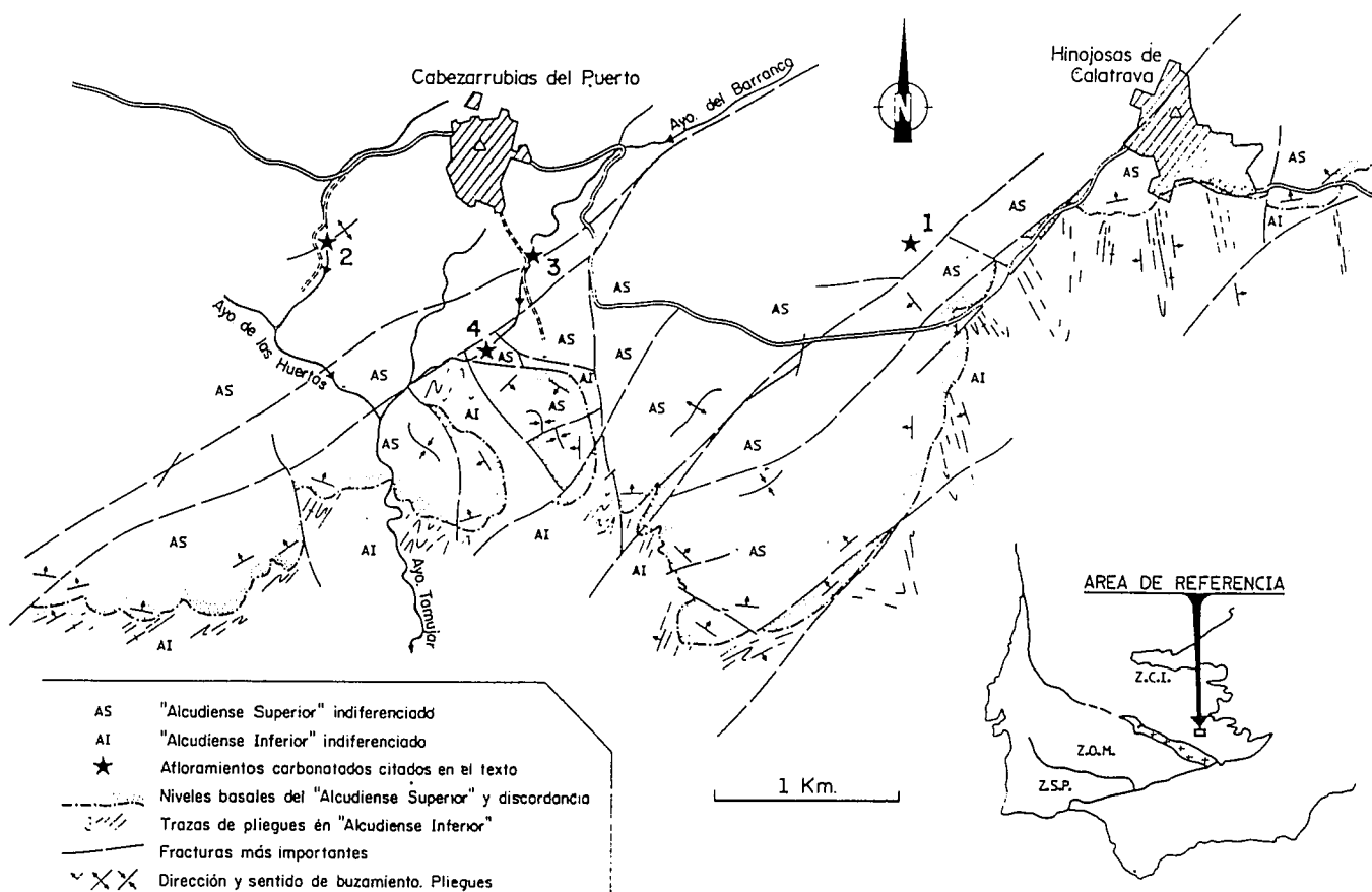
Fig. 1.—Esquema geológico del área Cabezarrubias-Hinojosas. Situación de los afloramientos.
