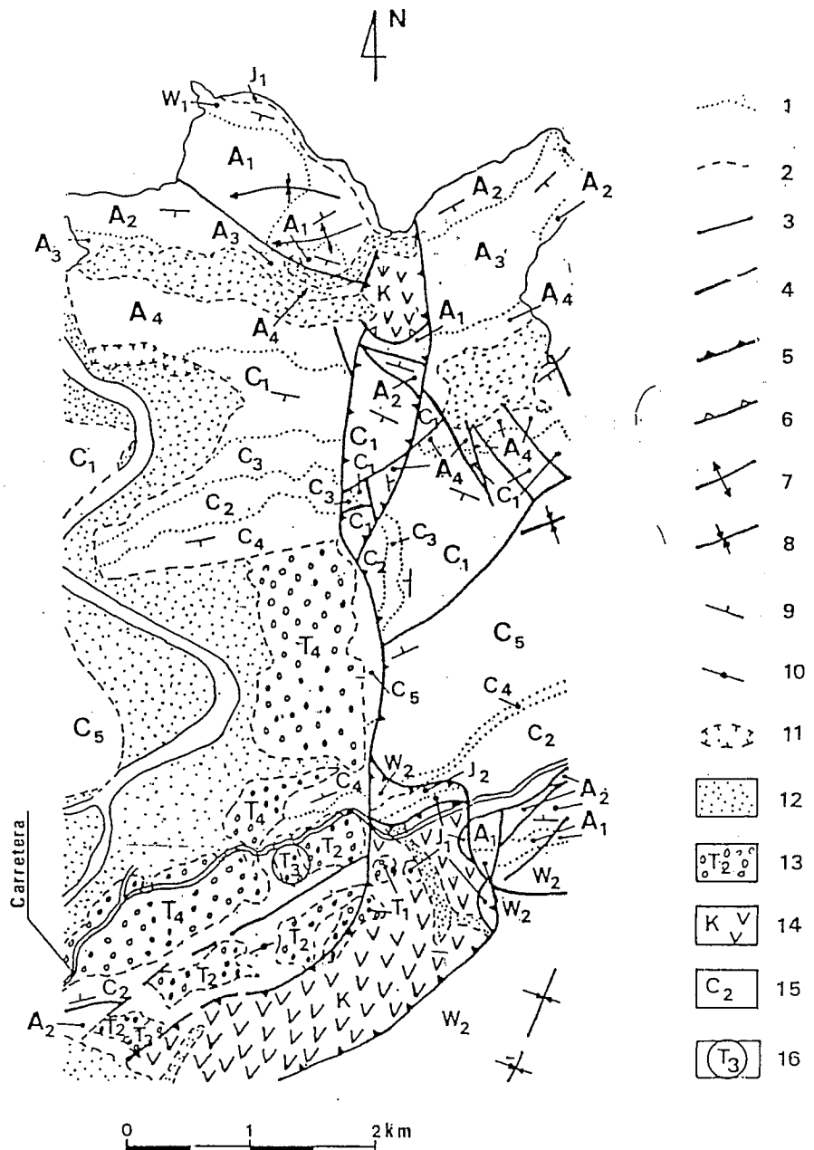
Fig. 1.—Esquema geológico de la zona de Polanco-Miengo (se- gún IGME, 1976):
