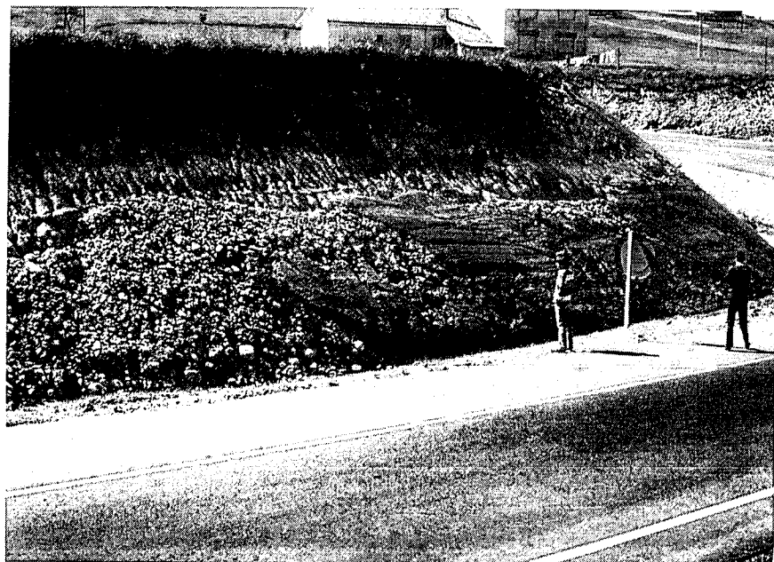
Fig. 2.—Fotografía (A) y esquema (B) mostrando el nivel inferior de cantos de la terraza, afectado por fallas inversas.
