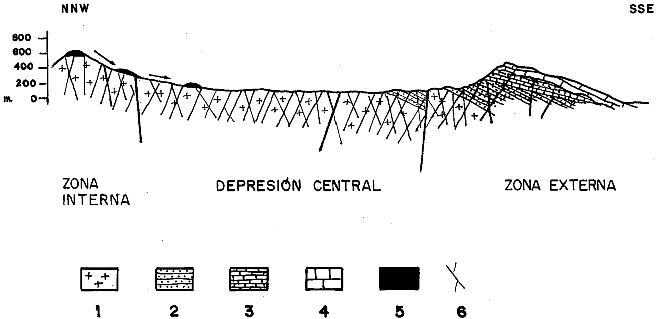
Fig. 1.—Corte tipo del Edificio Central de Fuerteventura. 1. Complejo Basal.—2. Serie I Inferior.—3. Serie I Intermedia.—4. Serie I Superior.—5. Serie I Tardía.—6. Diques.
