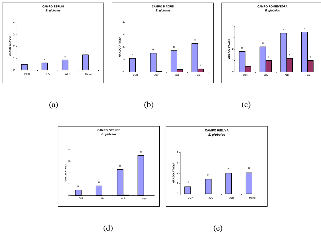
Fig. 2.- Valores medios de los grados de ataque producidos en la madera de albura (ALB), duramen (DUR) y juvenil (JUV), por los hongos xilófagos (H) y termitas (T) en los campos de ensayo de (a) Berlín, (b) Madrid, (c) Pontevedra, (d) Orense y (e) Huelva.
