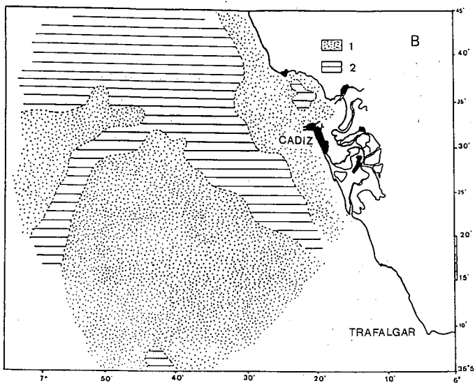
Fig. 2— Análisis Factorial (Modo-Q) de minerales. A) Representación gráfica de los valores (scores) de los minerales en los factores. B) Distribución de los factores (1.- Factor1: cuarzo-calcita; 1.- Factor2: filosilicatos-calcita).
