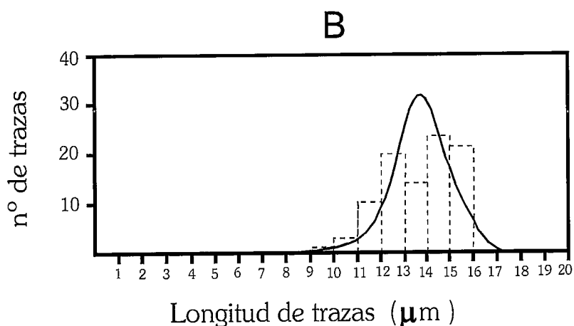
Fig.5.- Resultado de la optimización con el modelo Monte-Trax de Gallagher. A) Las 20 trayectorias temperatura-tiempo mas probables para la muestra GR-13; B) Distribución de longitudes de trazas confinadas fósiles correspondientes a la mejor trayectoria de enfriamiento.
