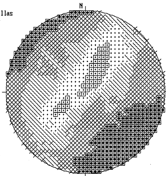
Fig. 3. Solución que aporta el método de los diedros rectos para las fallas de la estación de Bernuy. P: compresión; T: tensión.
