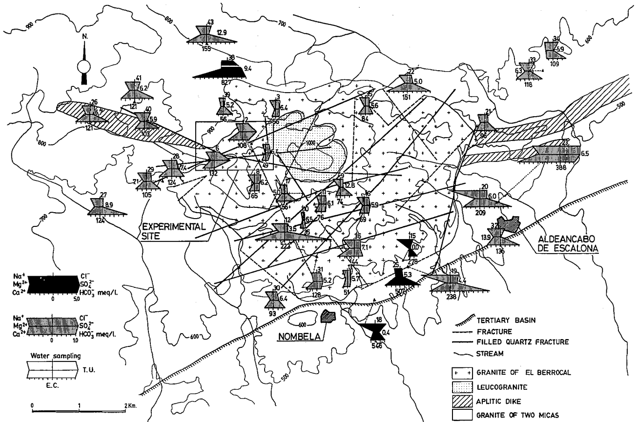
Fig. 1.- Esquema geológico del plutón del Berrocal, con los diagramas de Stiff modificados de los manantiales permanentes. Se indica también el contenido de tritio.
