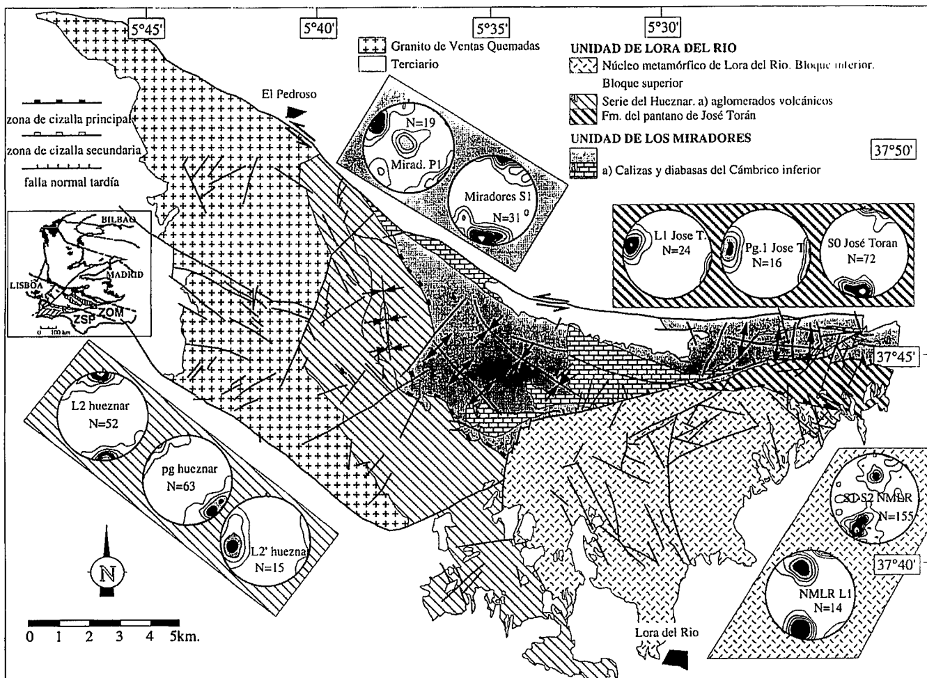
Fig. 1. Mapa geológico simplificado de la zona del núcleo de Lora del Río.
