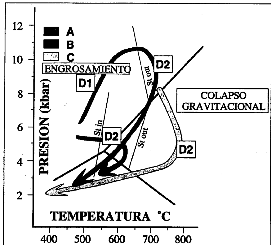
Fig. 2. Trayectorias P-T estimadas para: A) zona de la estauroлита en el bloque superior; B) rocas con asociaciones relictas Grt-Bt-Ky-Rt en el bloque inferior; C) rocas con asociaciones Grt-Crd-Bt-Fdk en el bloque inferior.
