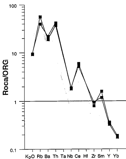
Fig. 5.- Spiderdiagramas normalizados frente al ORG (Pearce et al., 1984) para rocas del batolito de Los Pedroches. Cuadrados rellenos: diques traquiandesíticos; trama gris: variación de las composiciones para la unidad granodiorítica
