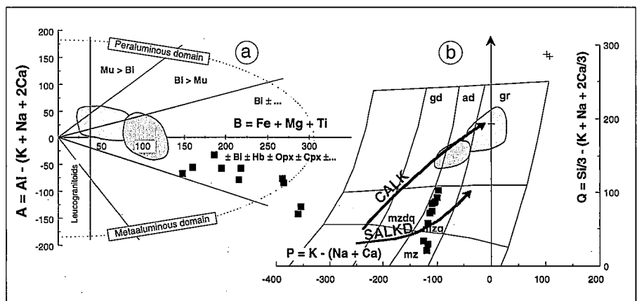
Fig. 3.- Diagramas A-B (a) y P-Q (b) (Debon & Le Fort, 1983) para los diques traquiandesíticos y las dos unidades plutónicas del batolito de Los Pedroches. Cuadros rellenos: diques traquiandesíticos; trama gris oscura: unidad granodiorítica; trama gris clara: unidad granítica.
