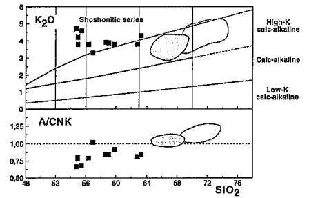
Fig. 2.- Diagramas K 2 O-SiO 2 (Peccerillo & Taylor, 1976) and A/CNK-SiO 2 para los diques traquiandesíticos y las dos unidades plutónicas del batolito de Los Pedroches. Cuadros rellenos: diques traquiandesíticos; trama gris oscura: unidad granodiorítica; trama gris clara: unidad granítica.
