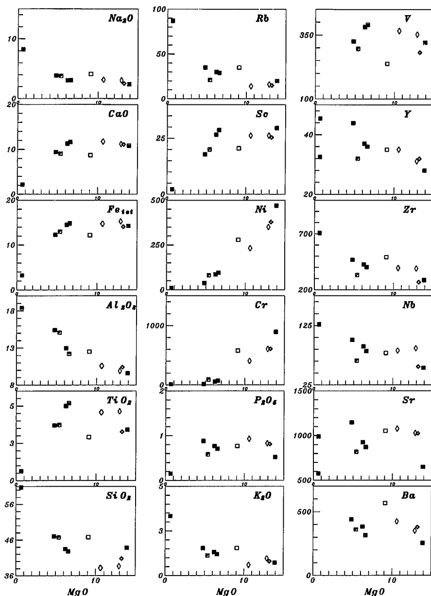
Fig.2.- Diagramas de evolución MgO - elementos. Rombos: Nefelinitas olivínicas de la Formación Angostura; cruz: Basanita de la Formación Angostura. Cuadrados: Resto de las rocas. Cuadrado vacío: Análisis n° 1905; Cuadrado semilleno: Análisis n° 1904.
