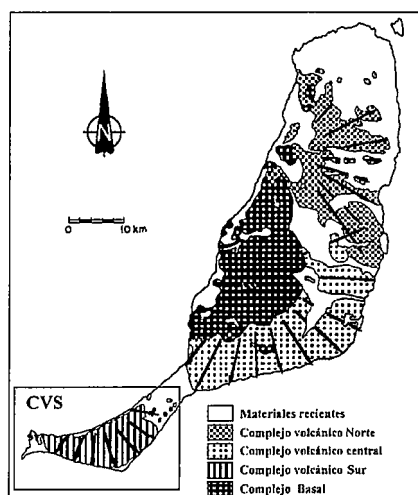
Fig.1.- Esquema geológico de los complejos volcánicos de la isla de Fuerteventura
