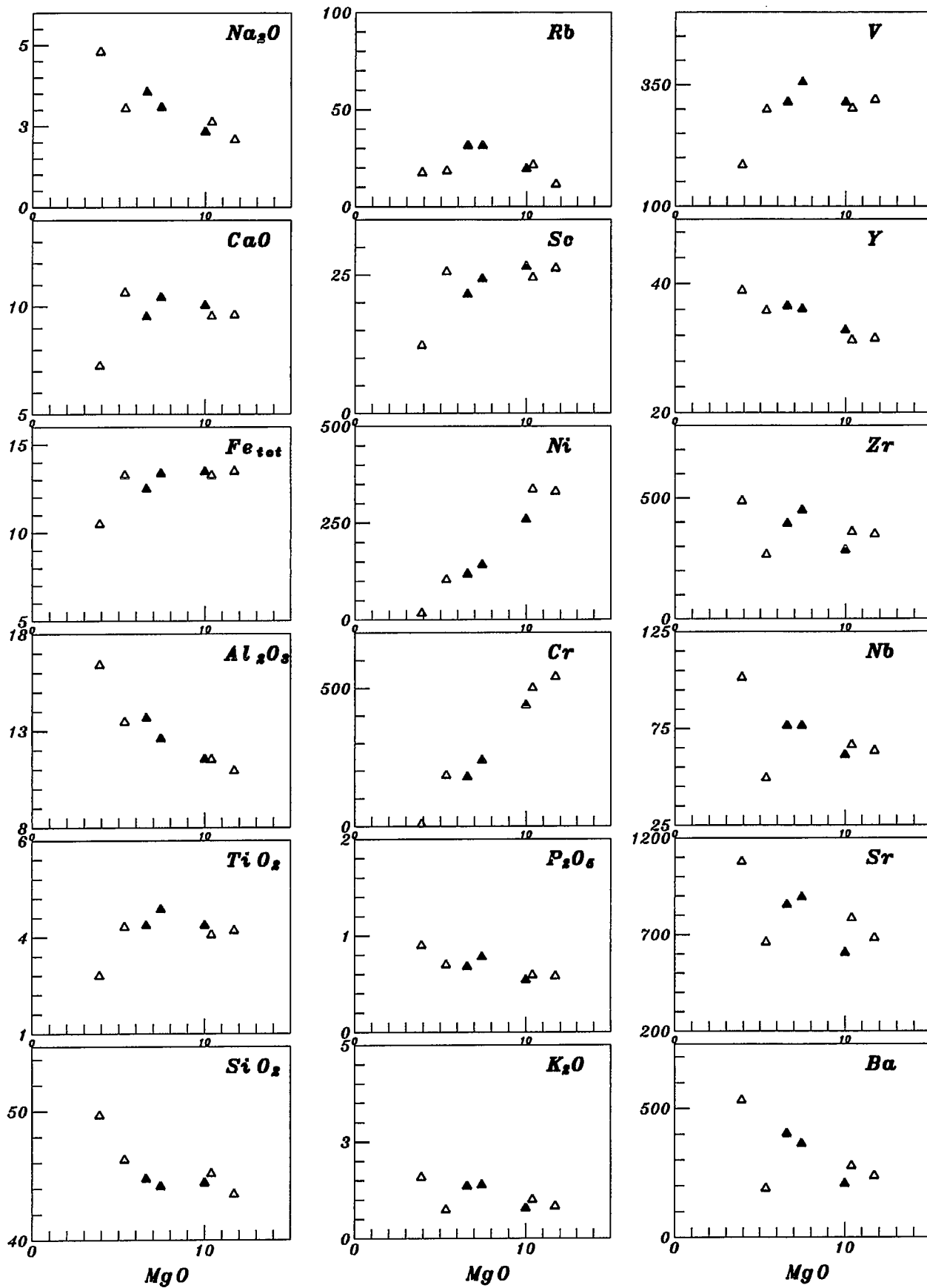
Fig.2.- Diagramas de evolución MgO - Elementos. Triangulo lleno: tramo bajo; Triangulo vacio: Tramo alto.
