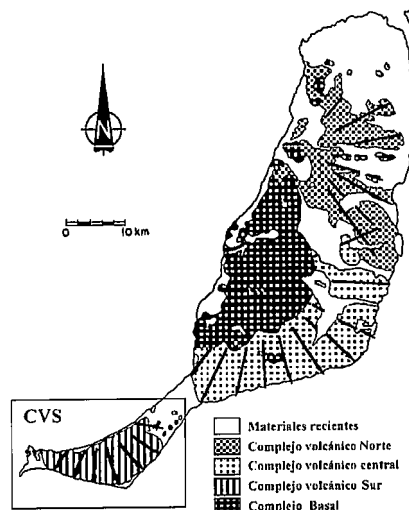
Fig.1.- Esquema geológico de los complejos volcánicos
