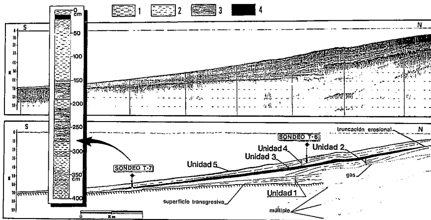
Fig. 2.- Perfil sísmico de alta resolución (3.5 kHz) en el delta del río Guadalhorce. Se muestran las unidades sísmica y la posición del sondeo T-7. 1: Arcilla gruesa, 2: Arcilla media, 3: Arcilla fina, 4: Arcilla muy fina.
