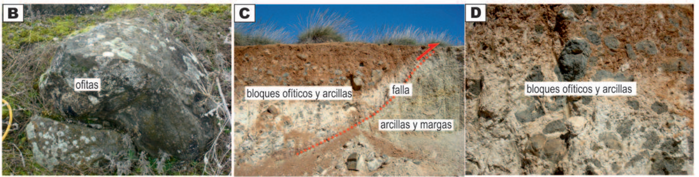
Fig. 2.- Interpretación de los perfiles de tomografía eléctrica realizados (X-X' e Y-Y'). La localización de los mismos aparece en la figura 1A. Se incluyen fotos tomadas en los afloramientos: afloramiento de ofitas (B); contacto entre los bloques ofíticos y margas cenozoicas (C); detalle de los bloques ofíticos (D). (Ver figura en color en la web).
