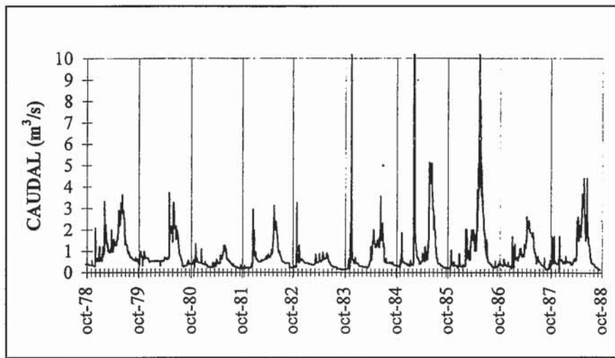
Fig. 2.- Hidrogramas analizados (ríos Monachil en Diéchar y Dílar en central eléctrica)
