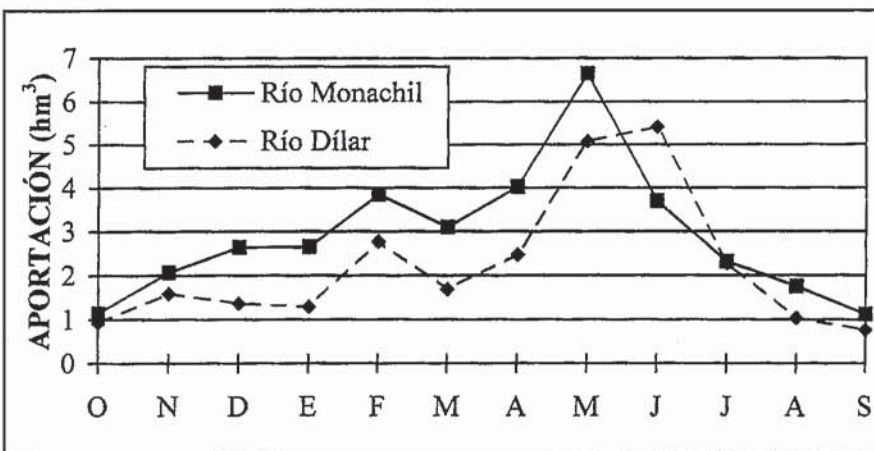
Fig. 3.- Hidrogramas medios mensuales del periodo considerado (ríos Monachil en Diéchar y Dílar en central eléctrica)
