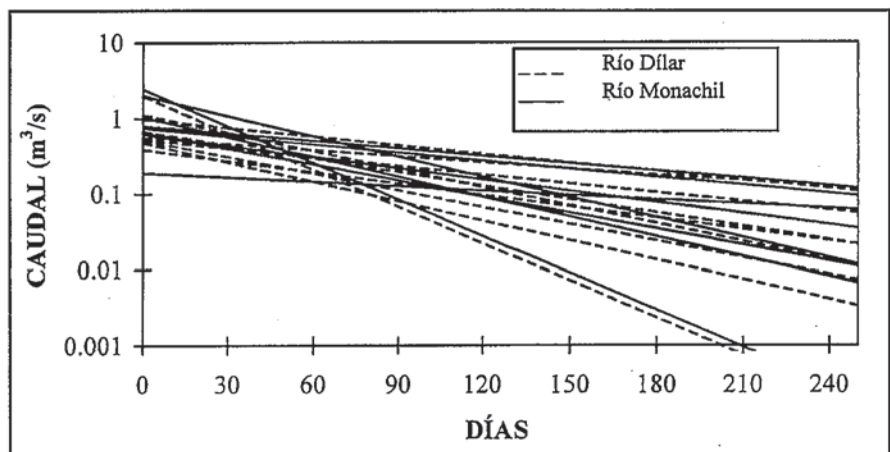
Fig. 4.- Curvas de agotamiento, a escala lognormal, de los ríos Monachil y Dílar (1978/79 a 1987/88)
